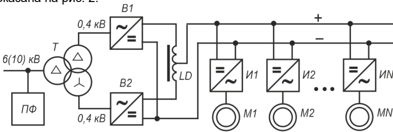
Рис. 2. Схема одной секции подстанции с шиной постоянного тока: Т – трансформатор; В1, В2 – выпрямители; LD – уравнивающий реактор; ПФ – пассивный фильтр; И1...ИN – инверторы напряжения с широтно-импульсной модуляцией
