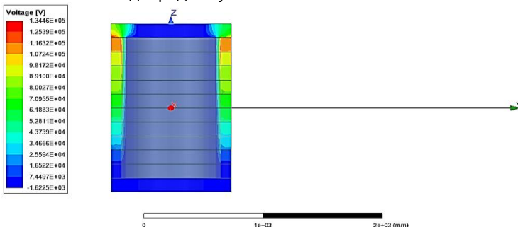
Рис. 2. Распределение потенциала вокруг обмоток
