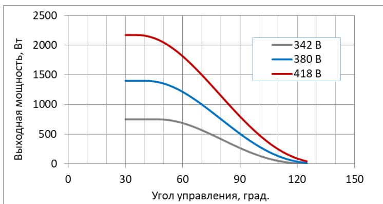
Рис. 2. Регулировочная характеристика
