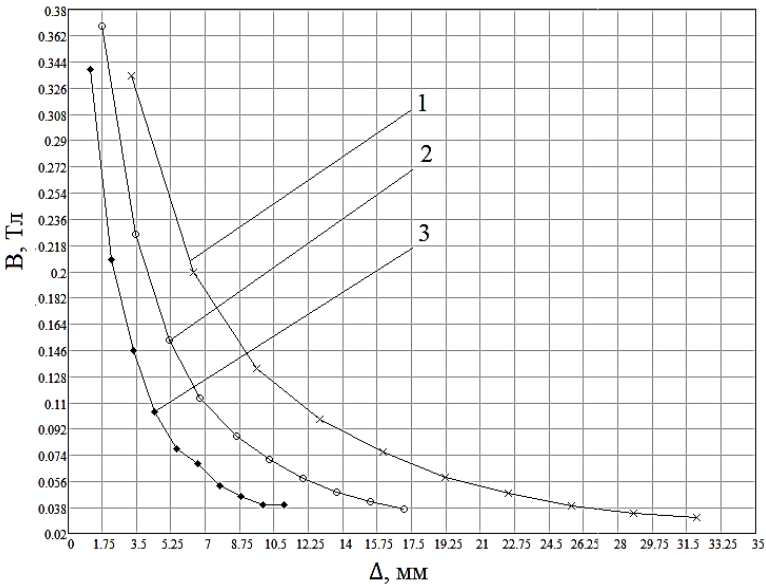
Рис. 3. Зависимости изменения магнитной индукции МЖДВ от расстояния между магнитами при 20°C: 1 – магнит K32×18×5; 2 – магнит K17,1×10×11; 3 – магнит K11×6×2,5
