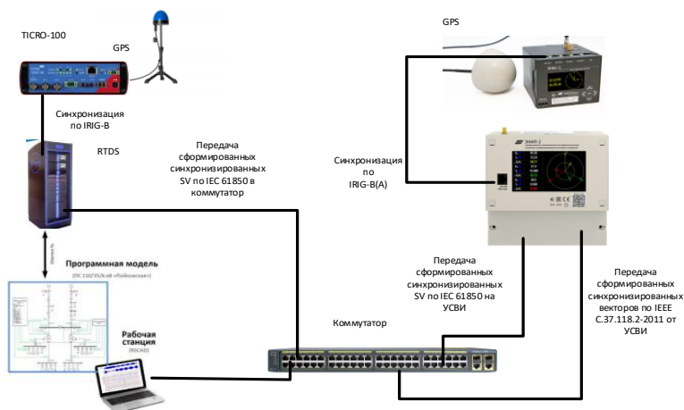
Рис. 1. Схема испытательной установки на базе ПAK RTDS
