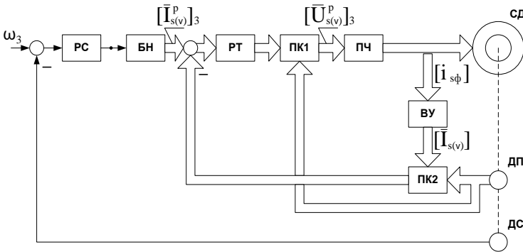
Рис. 2. Функциональная схема многоканальной САУ
