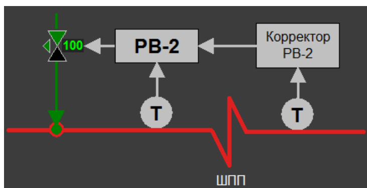
Рис. 3.14. Регулятор второго впрыска РВ-2
