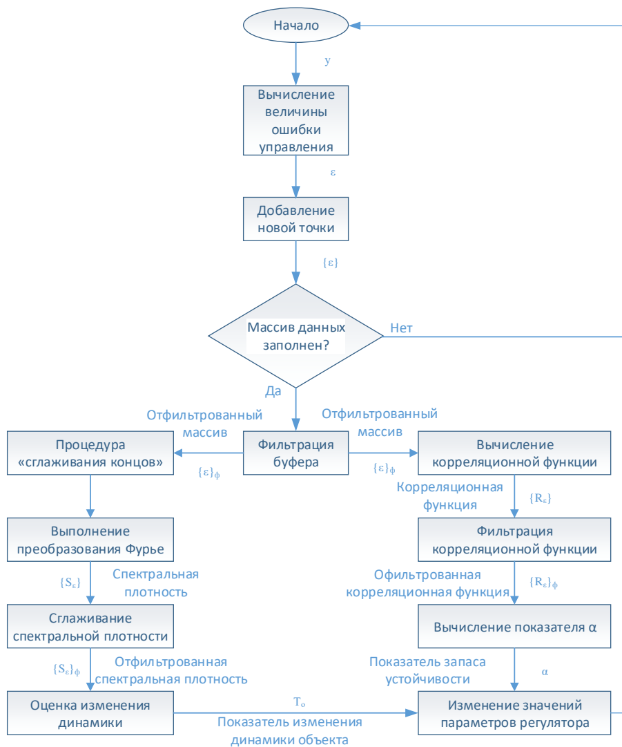
Рис. 2.17. Блок-схема алгоритма адаптивного управления
