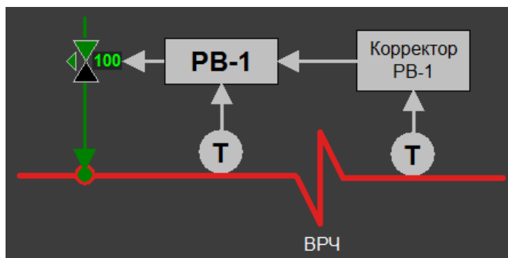
Рис. 3.14. Регулятор первого впрыска РВ-1
