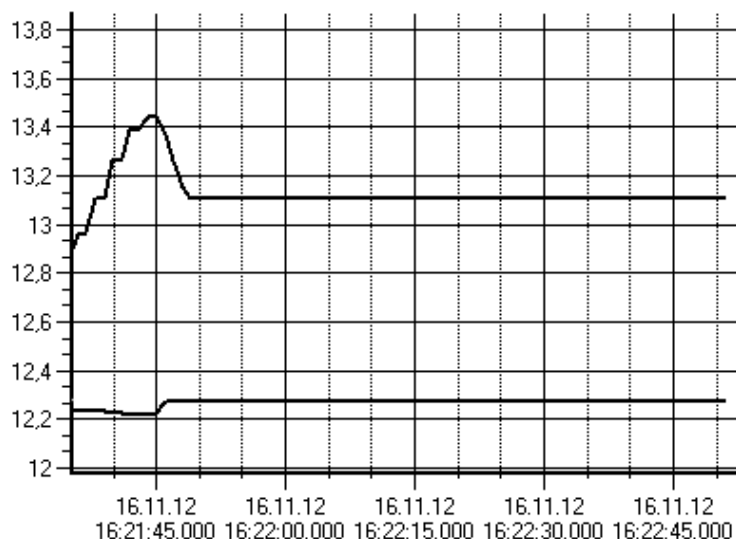
Рис. 3.26. Команда блокирования работы блока подстройки
