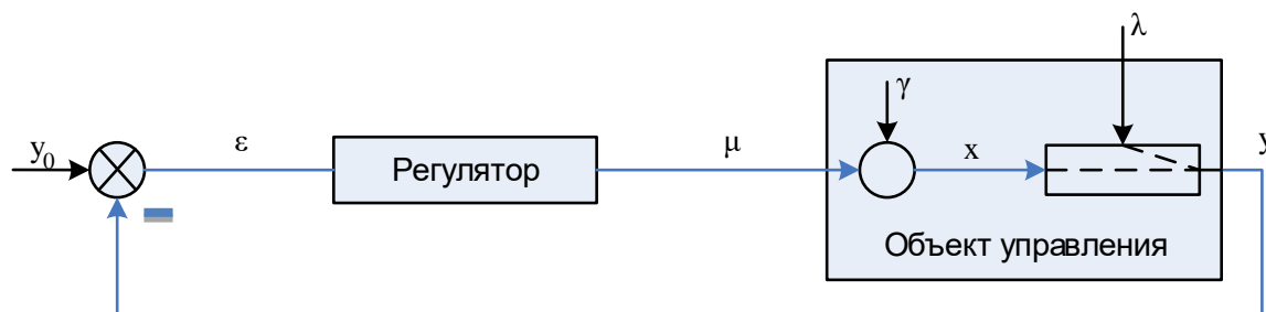
Рис. 2.2. Структура системы.
