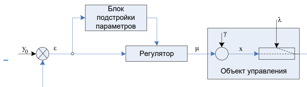
Рис. 1.3. Структура системы
