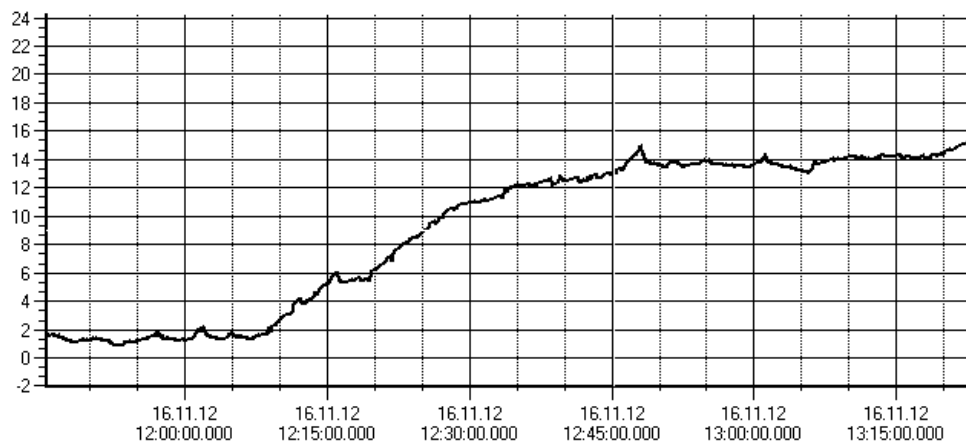
Рис. 3.18. Изменение коэффициента регулятора блоком подстройки
