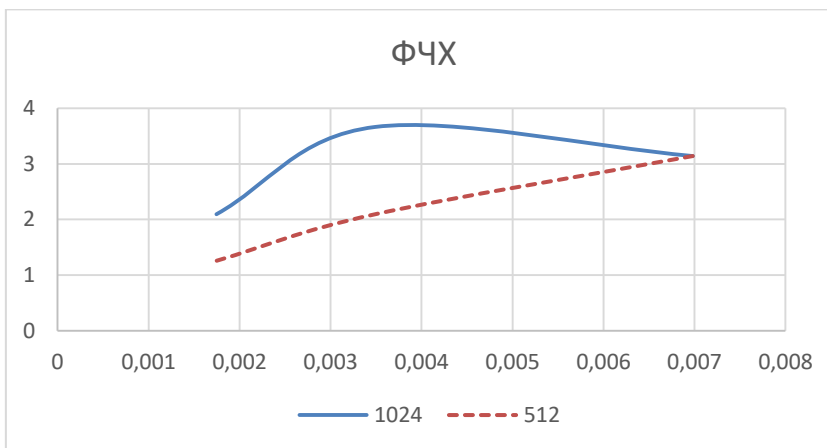
Рис. 4.5. Фазо-частотная характеристика
