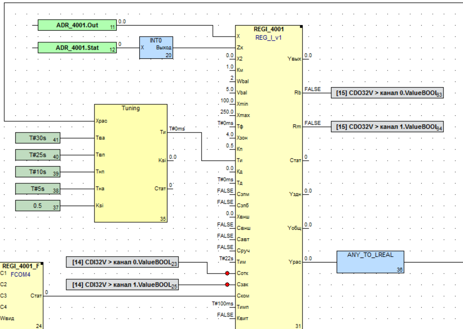
Рис. 3.5. Типовая схема совместного использования регулятора с блоком адаптивной подстройки
