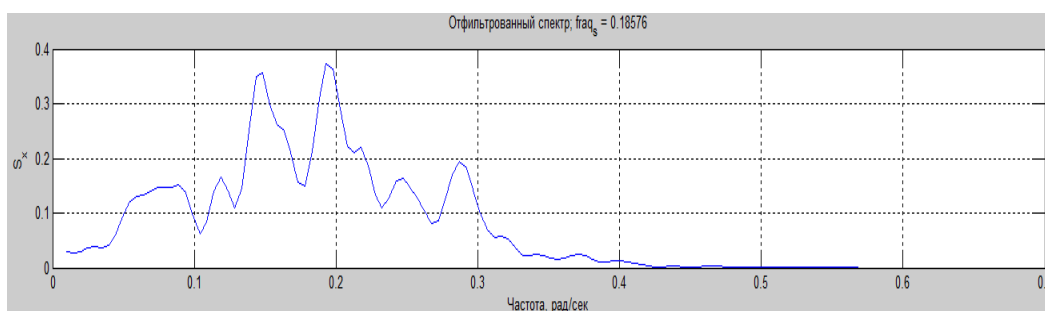
Рис. 2.11. Отфильтрованная спектральная плотность входного сигнала
