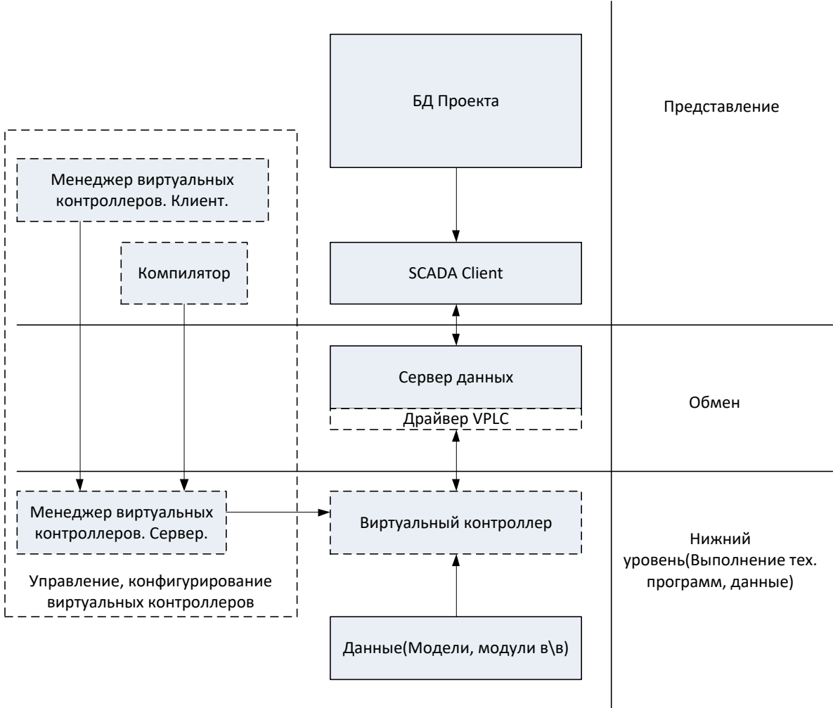
Рис. 3.7. Структура тренажера
