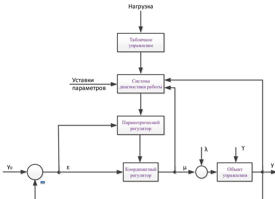
Структура системы
