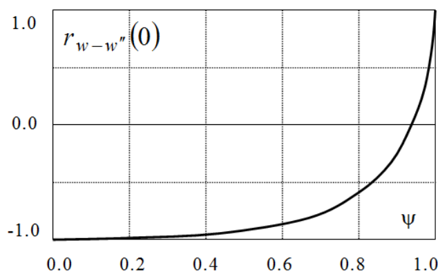
Рис.1.2. К оценке степени затухания процесса по взаимной корреляционной функции
