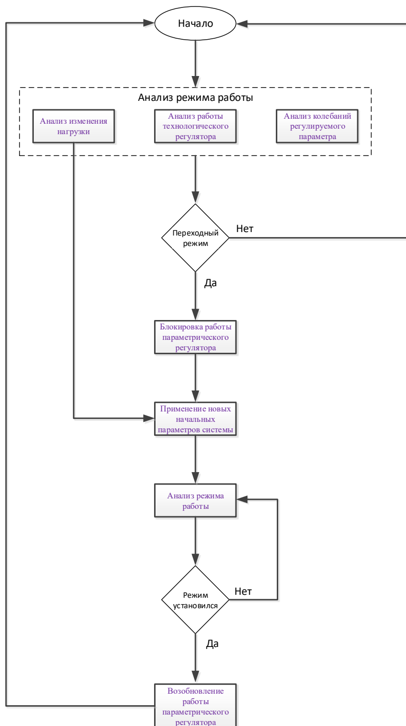
Рис. 3.3. Блок-схема алгоритма системы диагностики.
