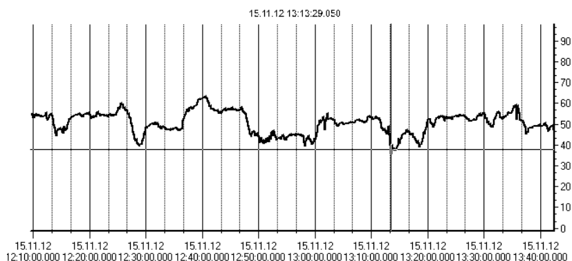
Рис. 4.21. Тренд значения перерегулирования при неизменных свойствах объекта управления
