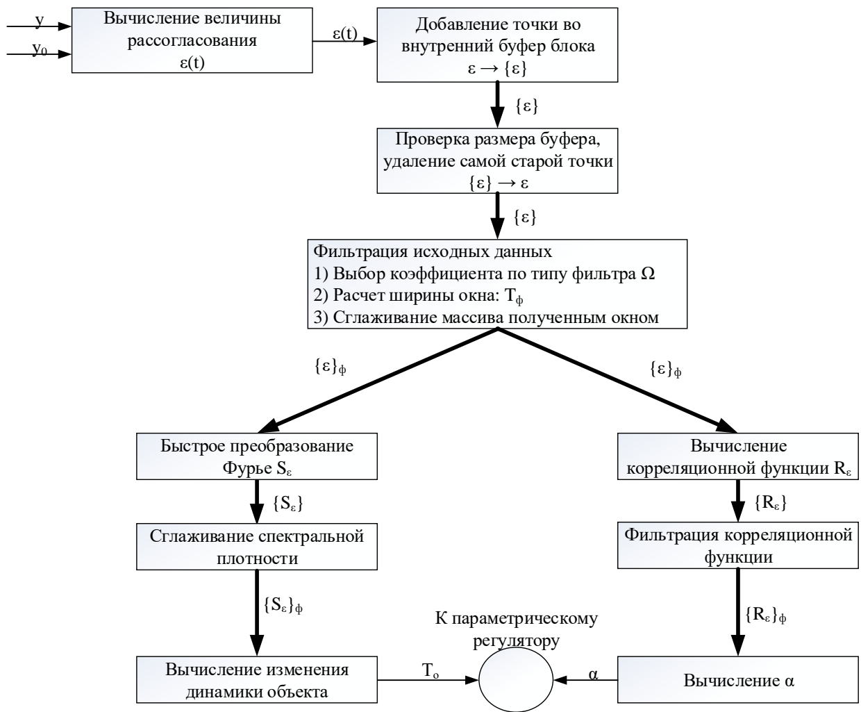
Рис. 2.18. Алгоритм адаптивного управления
