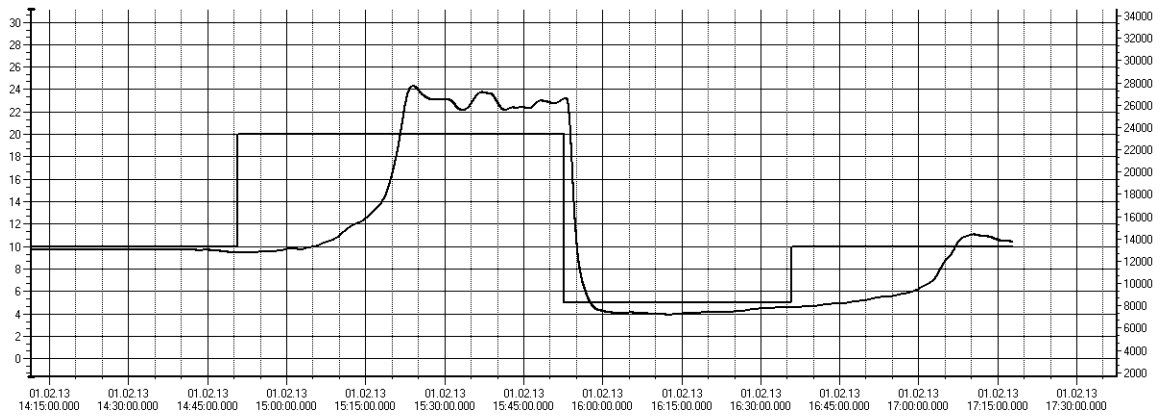
Рис. 3.24. Изменение времени дифференцирования при изменении постоянной времени объекта.
