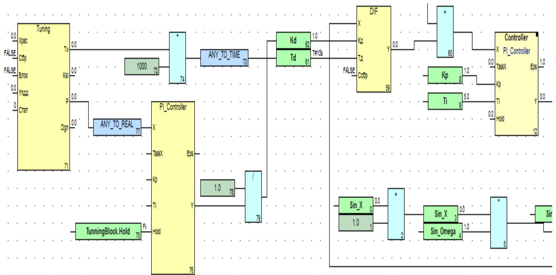
Рис. 3.23. Схема с дифференциатором
