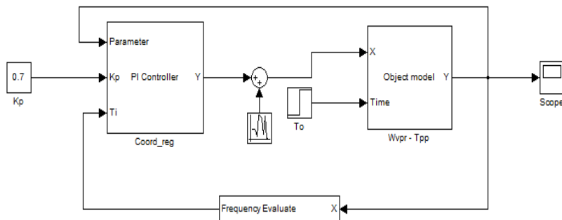
Рис. 2.24. Структура системы в программе MATLAB
