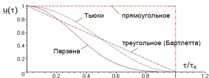
Рис. 2.12. Корреляционные окна
